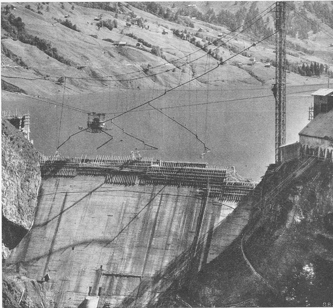
Abb. 1. Giessrinnen und Kabelkran zur Betonierung der Wäggital-Staumauer am 6. September 1924. (Phot. Wolf-Bender, Zürich.)
