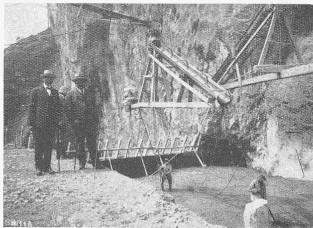
Abb. 4. Hölzerner Giessrinnen-Ausleger.
