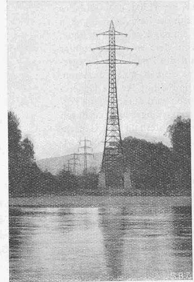
Abb. 8. Donaukreuzung von 330 m Spannweite.
