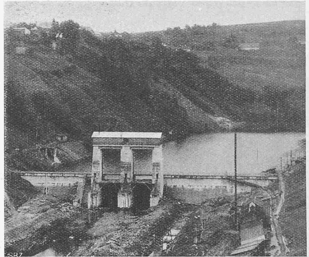
Abb. 3 und 4. Das Stauwehr des Kraftwerks Partenstein in der Grossen Mühl bei Langhalsen.
