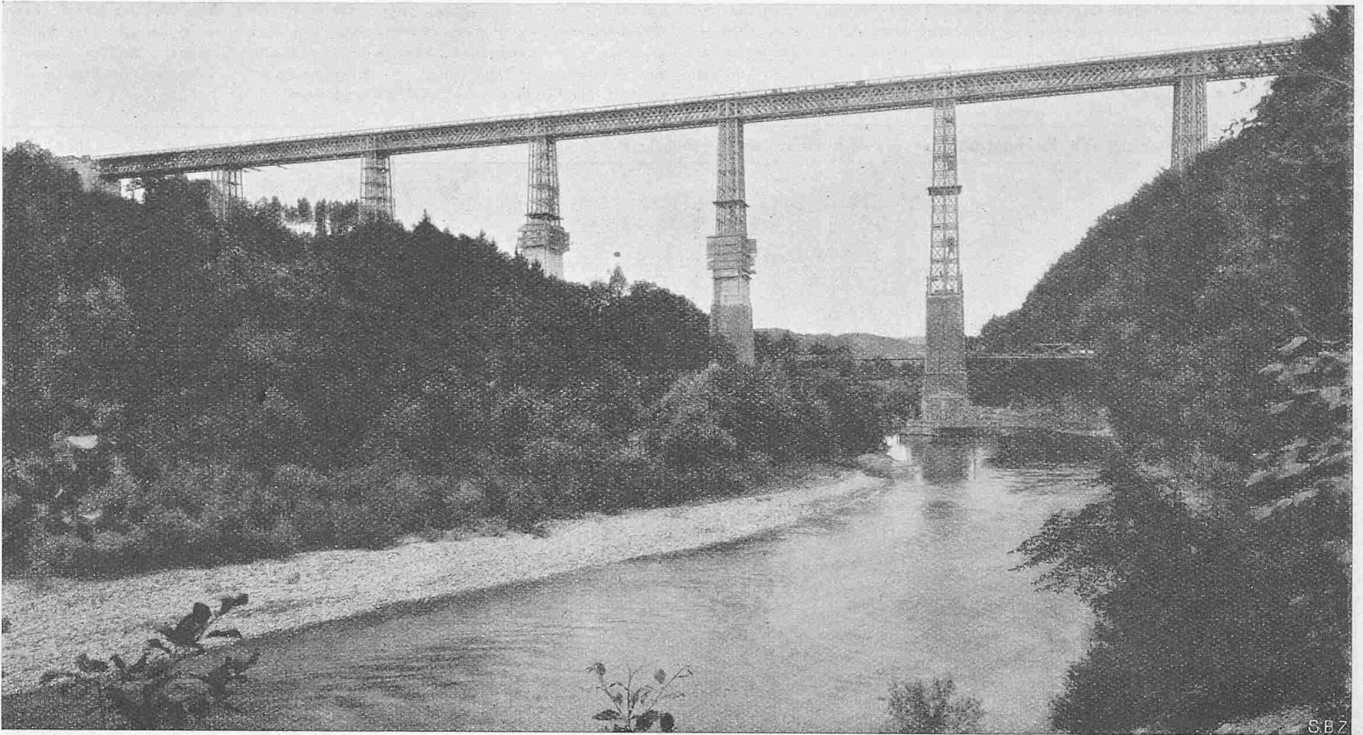
Abb. 2. Gesamtbild der alten Gitterbrücke. Beginn der Einbetonierung der eisernen Pfeiler über den gemauerten Sockeln (11. August 1925). Beim Flusspfeiler ist der alte Mauerwerksockel aus Molassequatern gut erkennbar.
