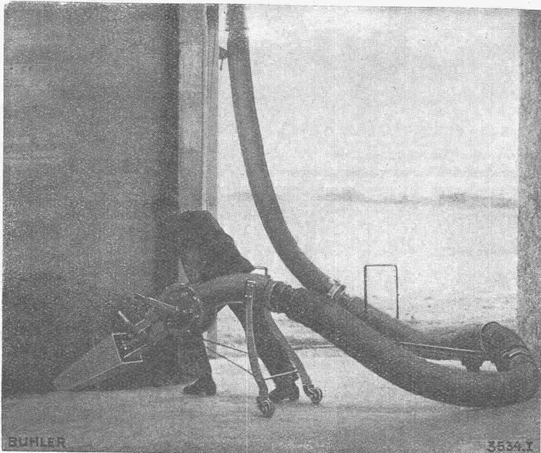
Fahrbare Spezialsaugdüse in einer Anlage für pneumatische Förderung von Erdnüssen (Arachides).
