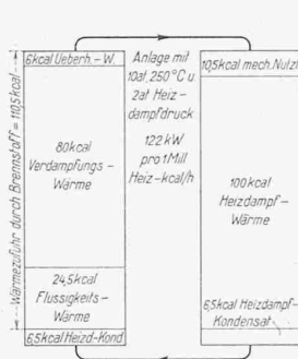
Abb. 10 und 11. Schemata des Kreisprozesses eines Heiz-Kraft-Betriebes für frühere Dampfverhältnisse 10 at, 250° C, 2 at Heizdampfdruck. 60 at, 450° C, 2 at Heizdampfdruck.
