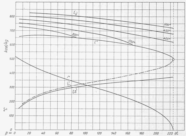
Abb. 6. Erzeugungswärme des Wasserdampfes für verschiedene Drücke und Temperaturen. i' Wasserwärme, r Verdampfungswärme, Ls Verdampfungstemperatur, i'' Wärmeinhalt des gesättigten Dampfes, iu Wärmeinhalt des überhitzten Dampfes.
