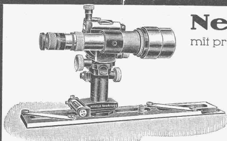
Kippregel Wild — \frac{1}{4} nat. Grösse
