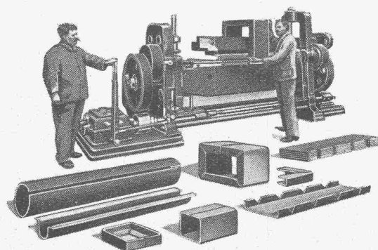
Universal-Abkant-Rund- und Kastenbiegmaschine D.R.P. und D.R.P.a.
