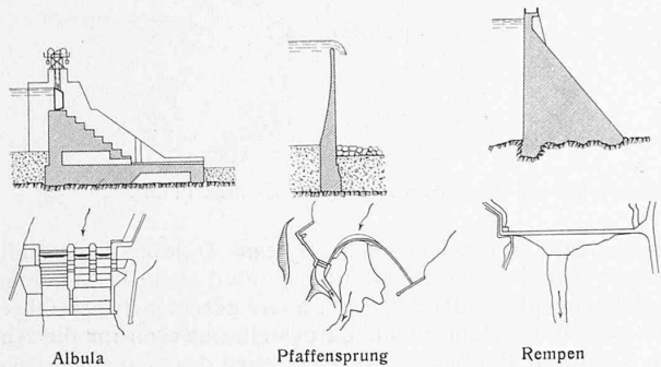
Abb. 7. Talsperren für Tagesausgleich. — Masstab 1 : 1600, bezw. 1 : 4000.
