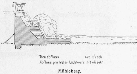
Abb. 4. Wehre mit Stauhöhen von 6 bis 25 m. — Schematische Darstellungen mit Angabe des Reguliervorganges und der Kolkwirkung. — Masstab 1 : 1400.
