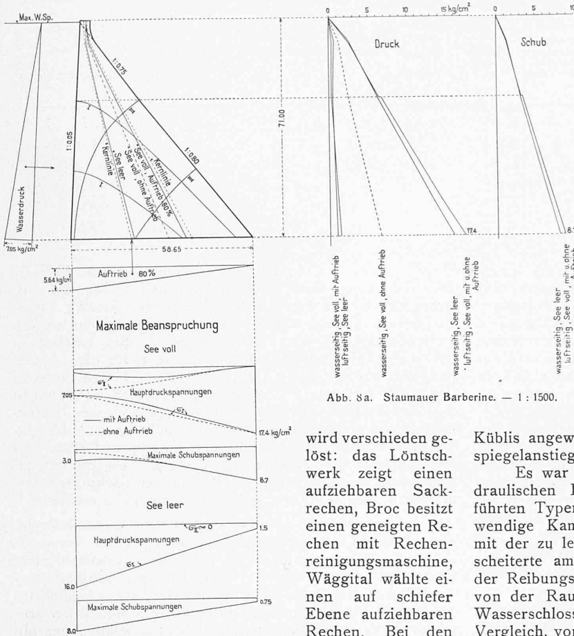
Verlauf der Drucklinien u. Hauptspannungen
