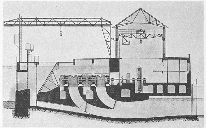
Rheinfelden. — Abb. 5. Maschinenhäuser. 1:500 (nach den farbigen Originalen clichéiert). — Augst.
