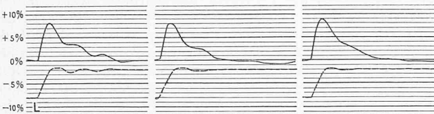
Abb. 9. Tachogramme der Versuchsserie L.
