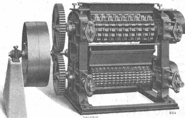
Doppelbrecher mit Zackenwalzen
