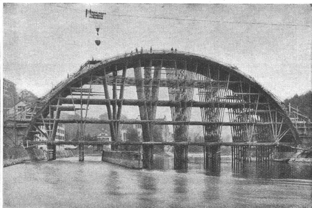
Lehrgerüst der Hochbrücke Baden, Spannweite 72 m.
