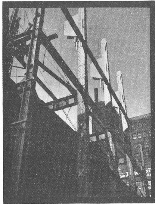
Abb. 10. Knotenbleche zur Befestigung der Gitterträger über den Bankettsäulen.
