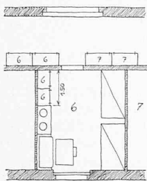
Grundrisse 1 : 200 der Schwesternzimmer zu zwei Betten nach Entwurf „Hors Concours“, nach Entwurf „Hospiz“.
