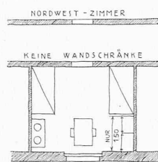
Grundrisse 1 : 200 der Schwesternzimmer zu zwei Betten nach Entwurf „Hors Concours“, nach Entwurf „Hospiz“.
