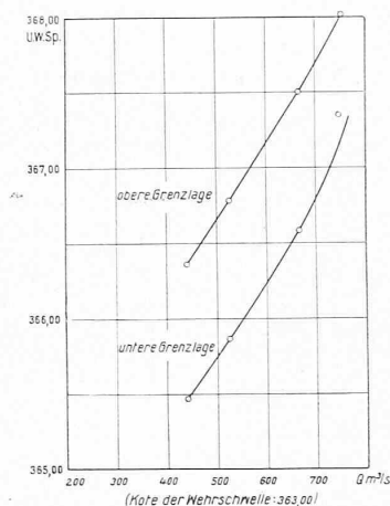
Abb. 6. Versuch mit der Wehrform W 4. Grenzlagen des Unterwasserspiegels für die Ueberlagerung des Wasserstrahls durch eine Deckwalze bei Abfluss ausschliesslich durch die Grundablasse.
