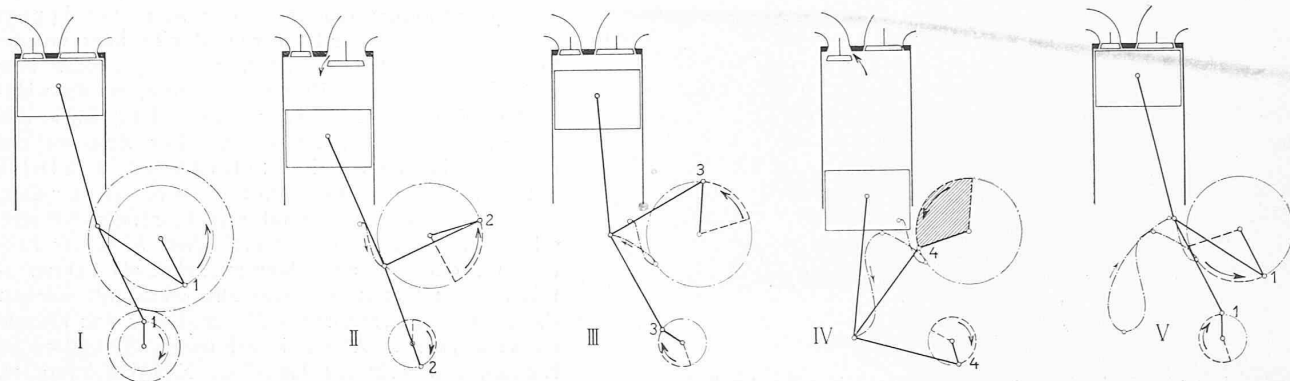
Viertaktmotor von Andreau mit ungleichen Hüten. — Schematische Darstellung der einzelnen Kolben-Endstellungen.
