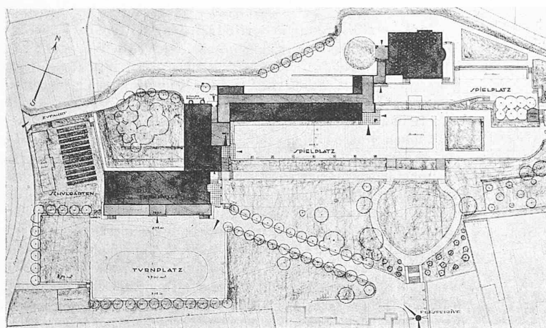
Lageplan. — Masstab 1 : 2000.
