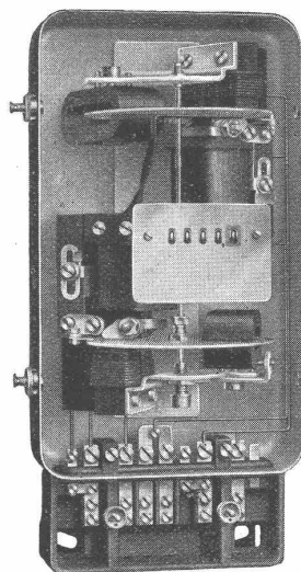
Drehstrom-Dreileiterzähler
