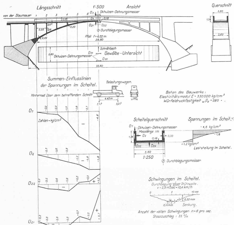
Abb. 7. Schräb Bach-Brücke des Kraftwerks Wäggit, Kanton Schwyz.
