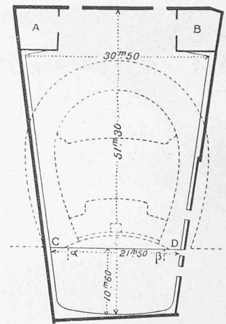
Abb. 1. Die Salle Pleyel in Paris. Grundriss. — Masstab 1 : 800. A B Treppen und Aufzüge, C D Rampe. (α β Bühnenöffnung der Grossen Oper.)
