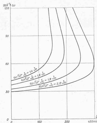
Charakteristiken, die zwischen \omega = 30 bis 60 für die Nutzbremse, zwischen \omega = 80 bis 120 zur Abgabe ungefähr konstanter Leistung dienen können.
