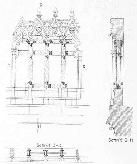
Abb. 5. Ersatz fehlender Glieder in der äusseren Trauf-Galerie. — 1 : 100.
