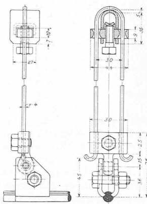
Abb. 16. Hängedrahtklemmen alter Bauart (Strecke Basel-Chiasso). Verschiedene Klemmen für Tragseil und Fahrdraht. 1:4.
