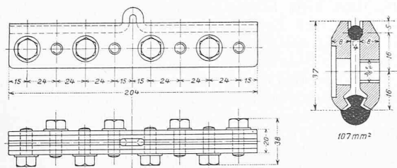
Abb. 15. Stossklemme für Fahrdraht von 107 mm 2 . 1:4. Querschnitt 1:2.
