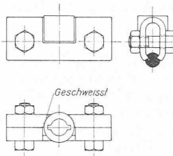
Abb. 19. Fahrdrähtklemme zum Spurhalterstab. 1:4.
