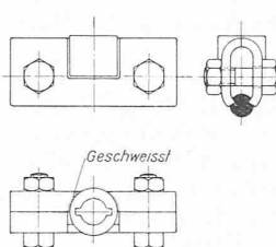
Abb. 19. Fahrdrahtklemme zum Spurhalterstab. 1 : 4.
