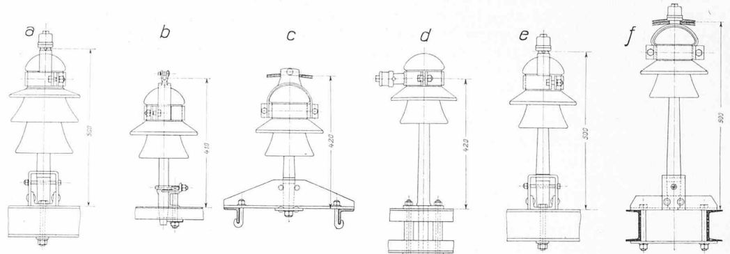
Abb. 24. Einfache Tragisolationen für die Tragseile, chronologisch geordnet. — Masstab 1:15.
