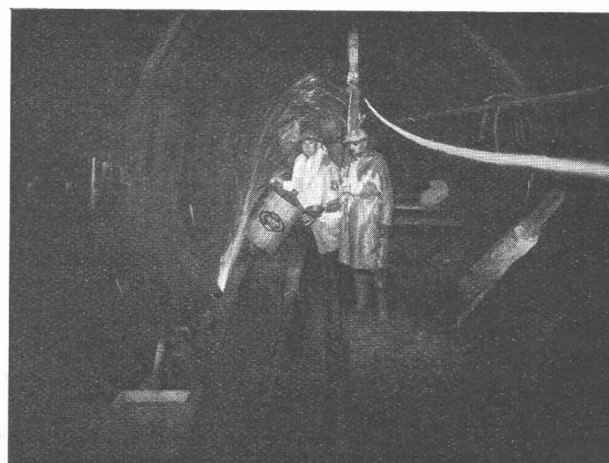
Sulgenbachstollen in Bern; Abdichtung starker Wassereinbrüche mit schnellbindender „SIKA“.
