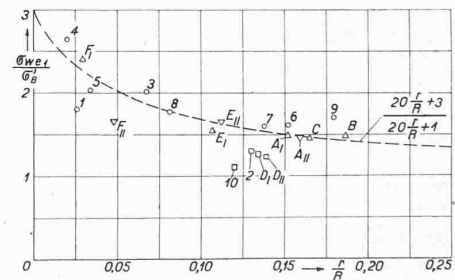
Abb. 11. Werte des Koeffizienten w in Funktion von r:R . Die Dreieckpunkte nehmen Bezug auf die Düsseldorf, die runden auf die Zürcher Versuche. Die Viereckpunkte betreffen elliptische Böden.
