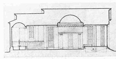
Entwurf Nr. 3. — Nordwestfassade, rechts Anschluss an das bestehende Bäderhaus. — 1:600. — Schnitt durch Trink- und Wandelhalle.
