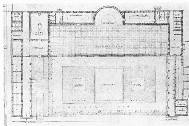
Oben: Grundriss 1:800.
