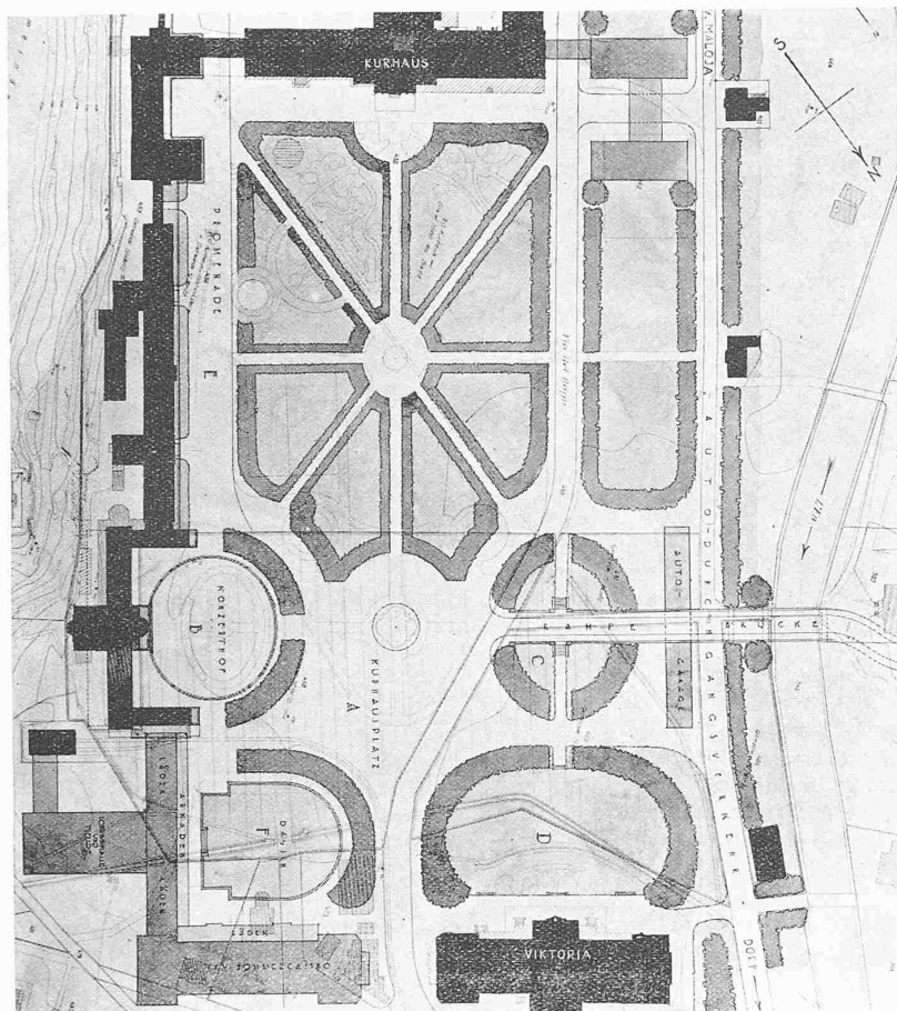
2. Rang (1300 Fr.). Entwurf Nr. 3. — Arch. Nic. Hartmann, St. Moritz. — Lageplan 1:2500.
