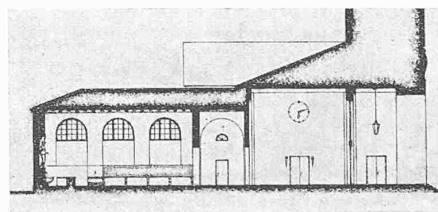
Schnitt durch die Gebäudemitte, darunter Grundriss. — 1 : 600.
