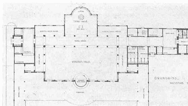
Schnitt und Grundriss 1 : 800.
