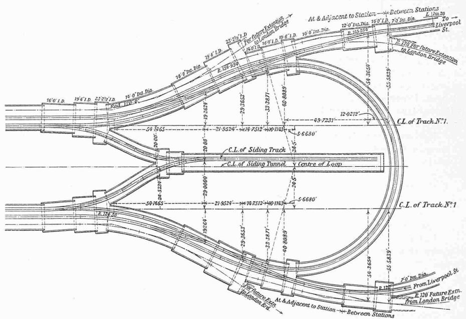
Abb. 3. Lageplan eines Stationsendes mit Schleife, Abstellgleise, Abzweigungen. — 1 : 600. (Nach „Engineering“).
