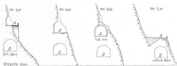
Abb. 23. Querprofile der obren Strasse. Einheitlicher Masstab dieser Querprofile 1:1000. Abb. 24 (unten). Querprofile der untern Strasse.
