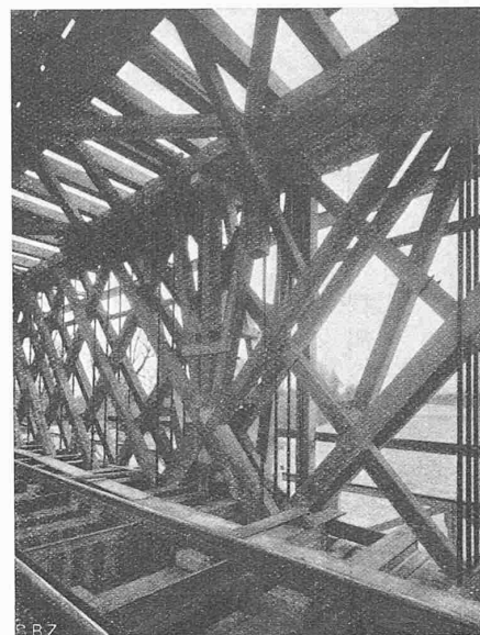
Abb. 10 Durchblick durch die alte Brücke, und Abb. 11 Ueberbau über den Pfeilern (bereits zum Abbruch vorbereitet durch Ab- und Einsagen einzelner Hölzer).
