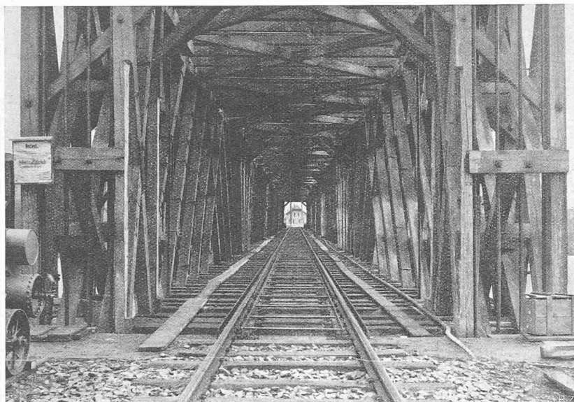
Abb. 10 Durchblick durch die alte Brücke, und Abb. 11 Ueberbau über den Pfeilern (bereits zum Abbruch vorbereitet durch Ab- und Einsagen einzelner Hölzer).
