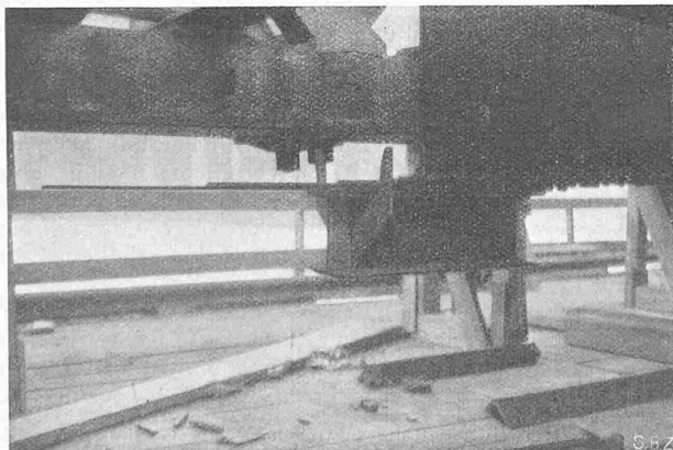
Abb. 24. Auffang-, Führungs- und Abstützkonsolle am Untergurtende des auskragenden Hauptträgers.
