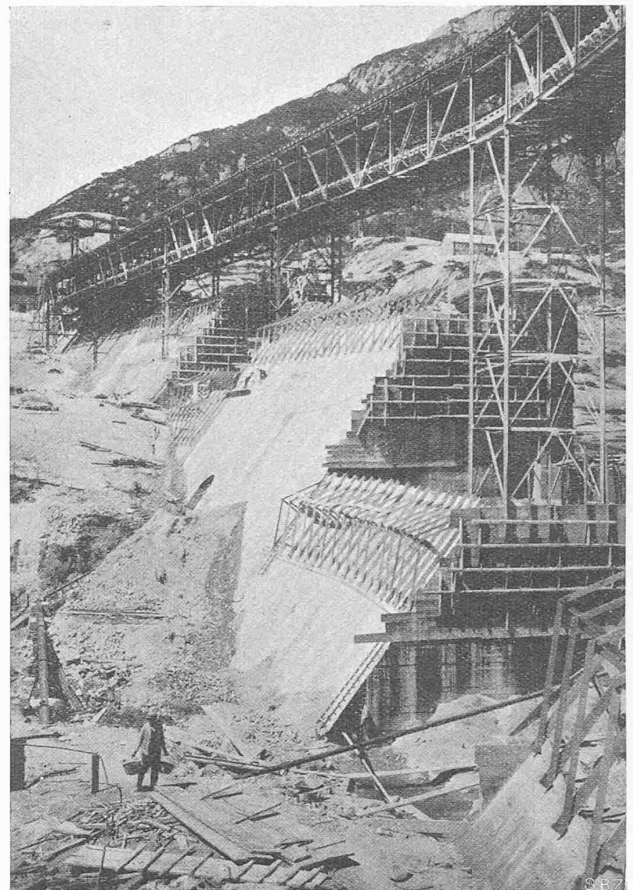
Abb. 12. Staumauer Gelmer, Luftseite gegen Norden gesehen.
