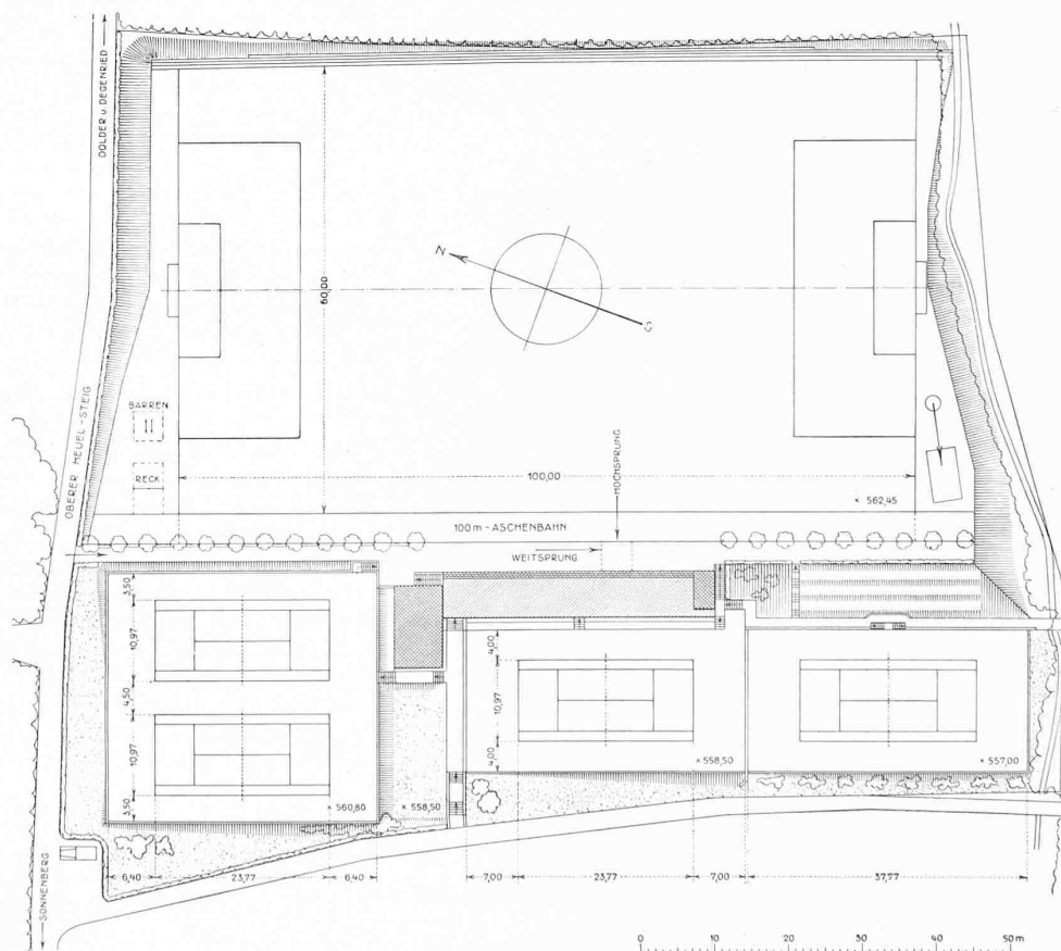
Abb. 1. Sportplatzanlage Sonnenberg, Zürich. — Lageplan, Massstab 1 : 1000.
