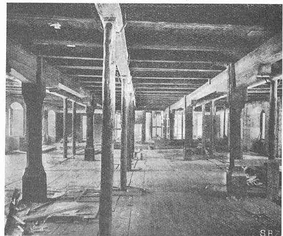
Abb. 6. Alter Holzständerbau im Obergeschoss.
