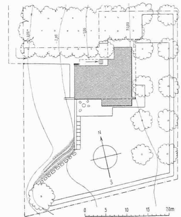
Abb. 1. Lageplan. — 1 : 800.
