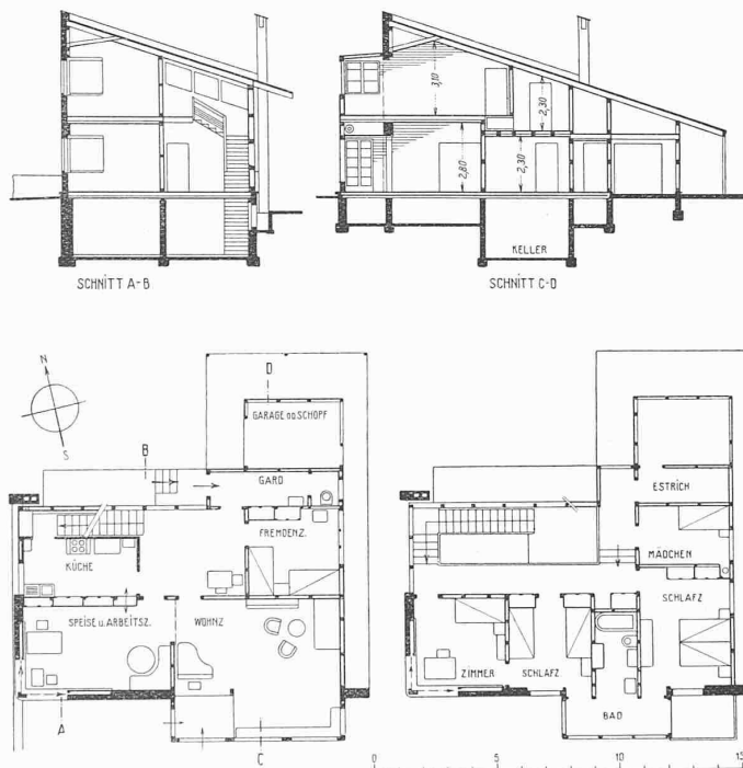
Abb. 2 bis 5. Grundrisse und Schnitte. — Masstab 1 : 300.
