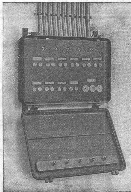
Lichtinstallationskasten (geöffnet)
