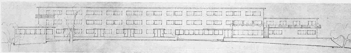
2. Rang, Entwurf N. 6. Arch. E. & O. Oeschger, Zürich. Südfassade, Schnitte und Grund- risse. — Masstab 1:600. Lageplan 1:2000.
