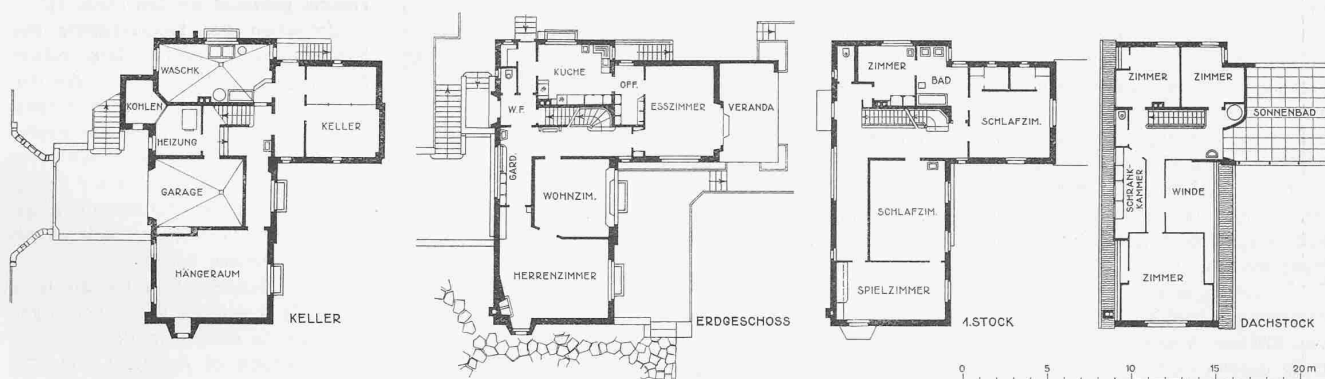
Abb. 4. Grundrisse, Masstab 1 : 400.
