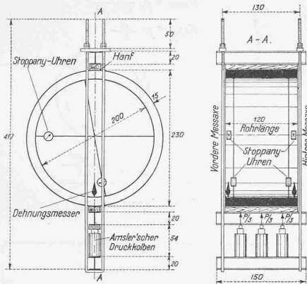
Abb. 9 und 10. Allgemeine Anordnung und Ergebnisse der Scheitelbelastung mit 22,4 t eines 1,20 m langen Rohrstückes von 200 m l. W. (Sohle innen).
