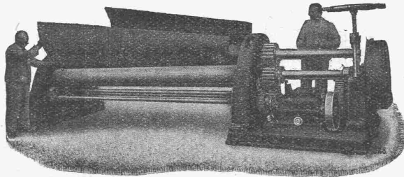
Vierwalzen-Blechrund- oder Biegemaschine
