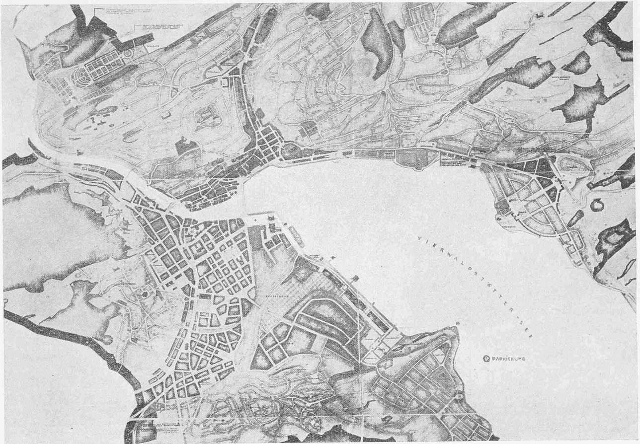
2. Rang (2800 Fr.), Entwurf Nr. 7. Verfasser: Möri & Krebs, Architekten, Luzern. — Uebersichtsplan 1:25 000.
