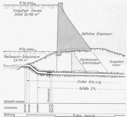
Abb. 4. Vertikalschnitt in der Axe des Umleitstollens, 1:1500; Gestrichelt: Schnitt im Talweg.
