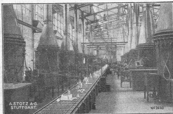
Bandförderanlage
