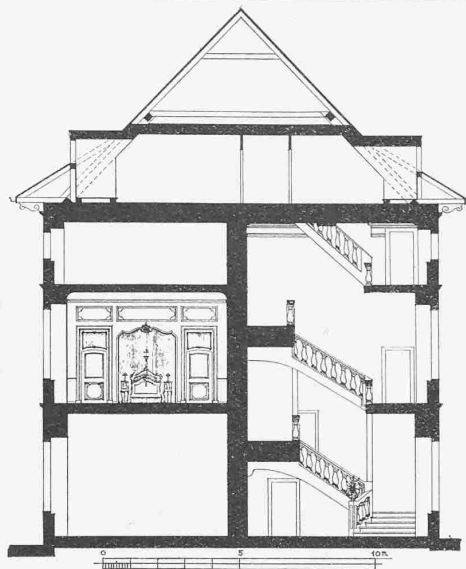
Abb. 9. Schnitt. — 1:250.
