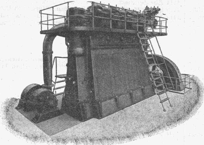
1150 PSe „S. L. M.-Winterthur“-Dieselmotor mit Büchi-Abgas- turbinaufladung
