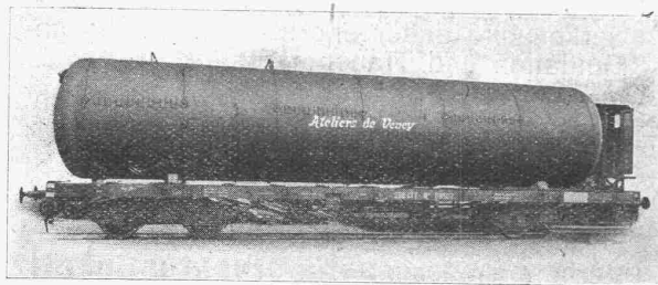
Gasbehälter, vollständig geschweisst. Innerer Druck : 5 Atm. • Inhalt : 100 m³.
