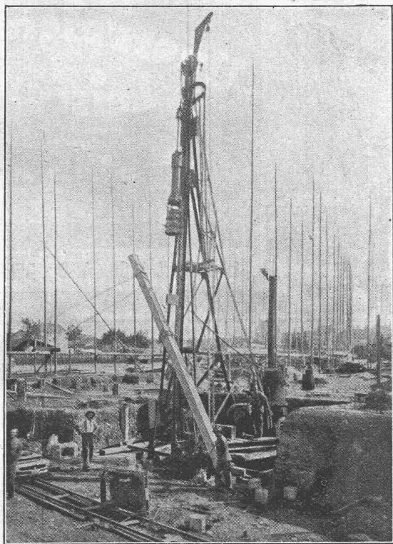
Foundation Wohnhäuser A. B. Z. Seebahn-Kanzleistrasse, Zürich 4 mittelst Eisenbetonpfählen System „Züblin“.
