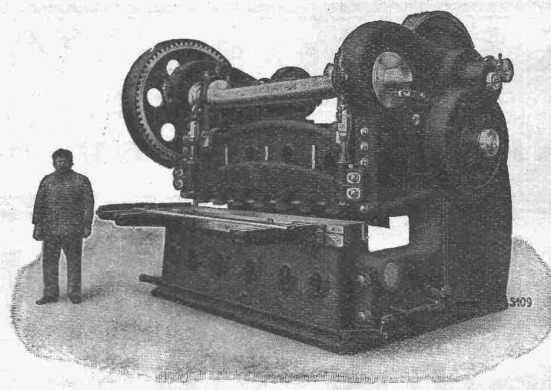
Kurbel-Blechtafelschere
