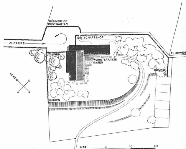
Abb. 1. Lageplan. — Masstab 1 : 800.
