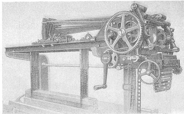
Abb. 17. Tiefliegende Doppelhub-Schaftmaschine mit Hubexzentern.
