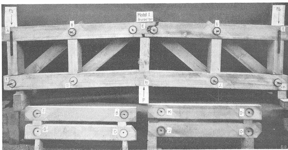
Abb. 15 (unten). Fachwerk-Modell II, Bruchlast 1310 t.
