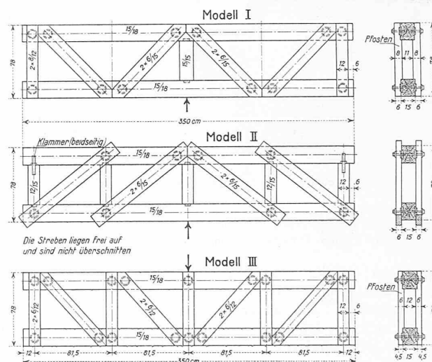
Abb. 13. Fachwerk-Modelle I bis III. — Masstab 1 : 50.
