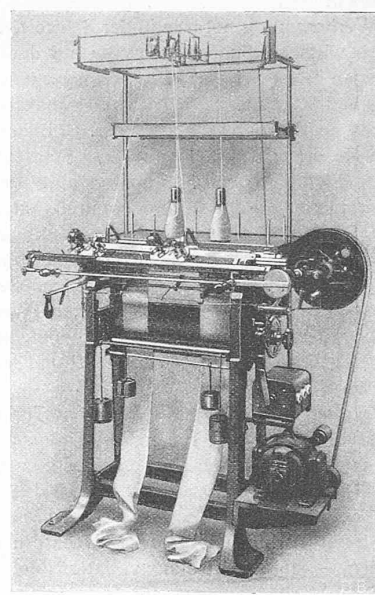
Abb. 29. Motorangetriebene Bandstrickmaschine.
