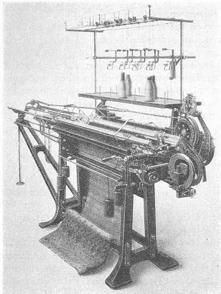
Abb. 26. Halbautomatische Jacquard-Strickmaschine.
